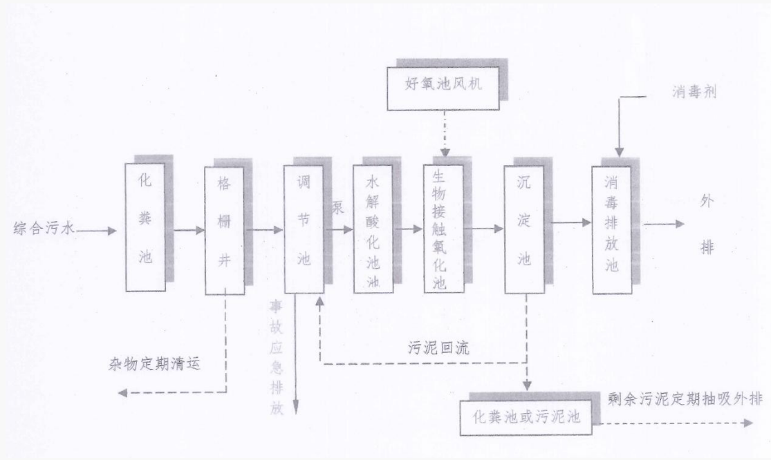
图3-3 污水处理工艺图
